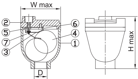
DN25 DIMENSION 尺寸表
